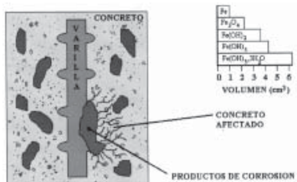
Fig. 1. Efectos de la corrosión del acero en el concreto armado.
