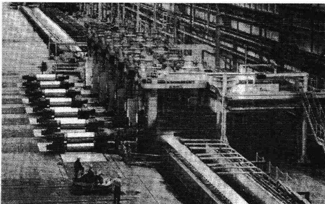
Figura 2.4.- Esta vista muestra la salida del molino continuo. También se observan rodillos de trabajo nuevos, alineados y listos para un cambio general de rodillos 3 .
