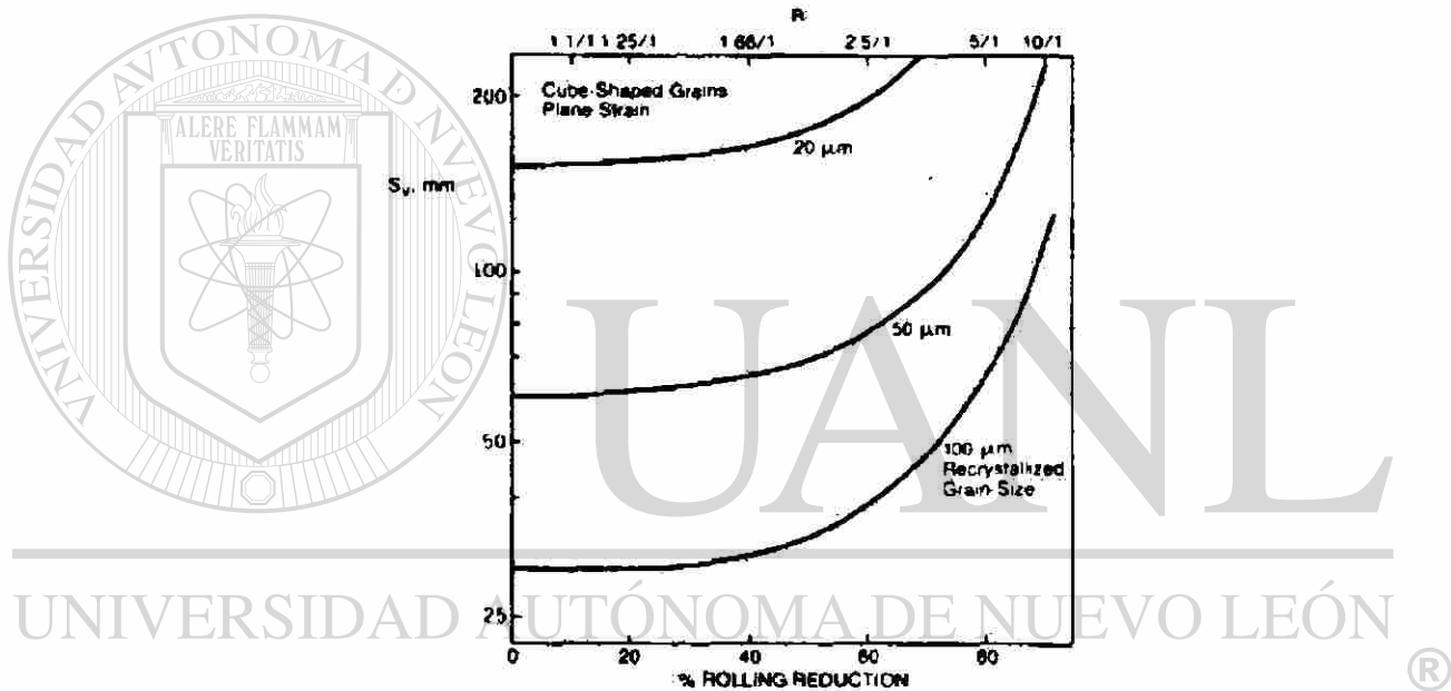
Figura 3.4.- Efecto del proceso de laminado sobre Sv en granos de austenita 5 .
