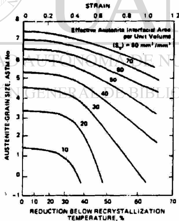
Figura 3.5.- Variación de Sv con la deformación por debajo de la temperatura de recrystalización 4 .
