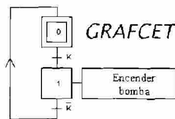
Figura 7.8 Etapa de salida de una transición.
