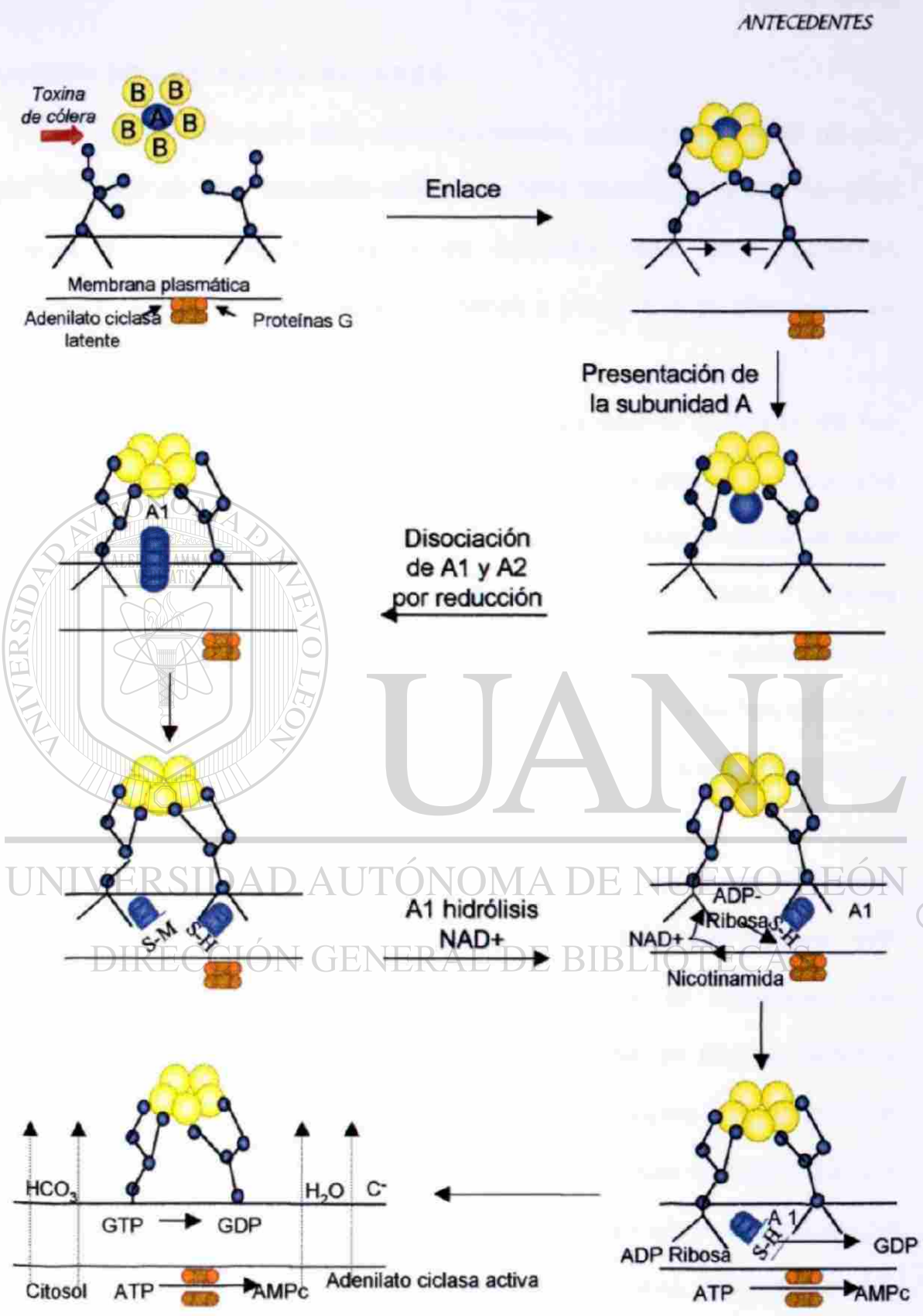
Fig. 1) Modo de acción de la toxina de V. cholerae
