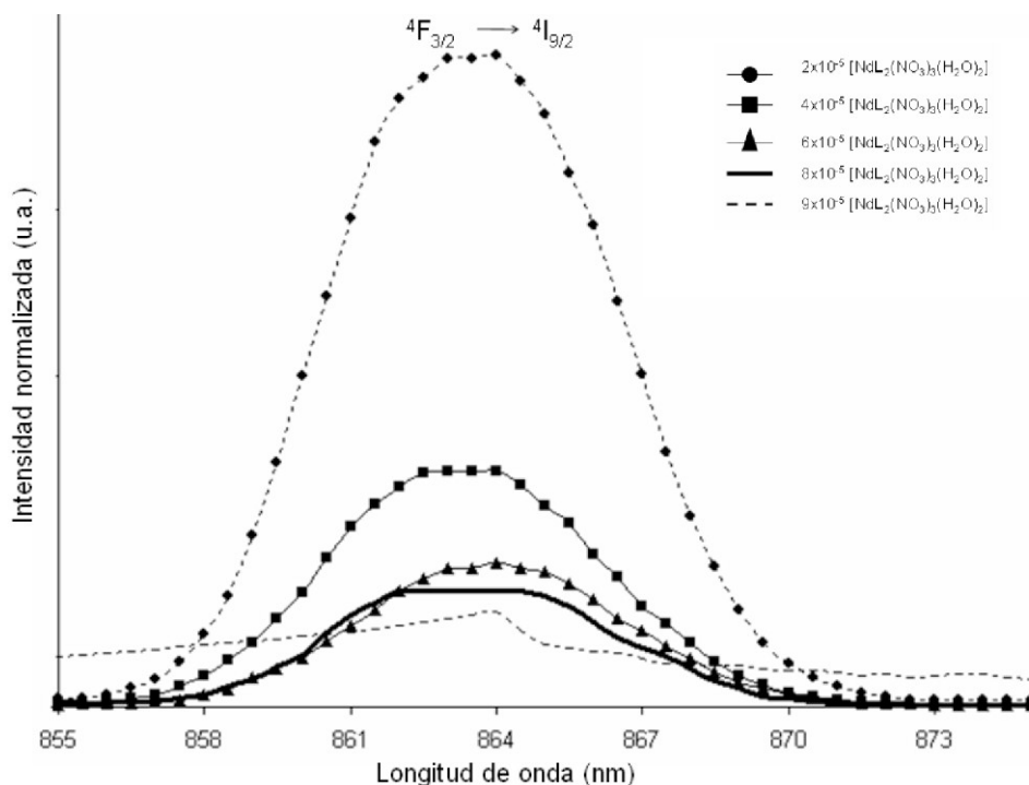
Figura 2. Espectros de emisión de las disoluciones de [NdL_2(NO_3)_3(H_2O)_2] .
