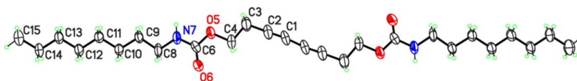
Figura 1. Representación ORTEP de una molécula del compuesto 1 , con elipsoides de desplazamiento para C, N y O a 30% de probabilidad. La unidad asimétrica está constituida por los átomos C1...C15, y los átomos no etiquetados se generan por un centro de inversión cristalográfico.
