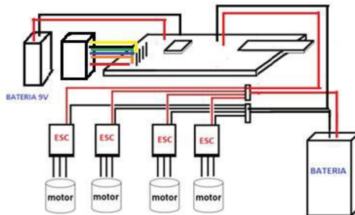
Figura 1 Esquema de conexión
